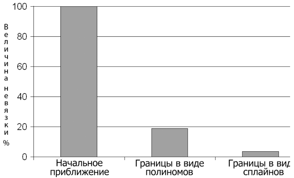
4. Значения общей среднеквадратичной невязки по всем присутствующим годографам ВСП, выраженные в процентах.
