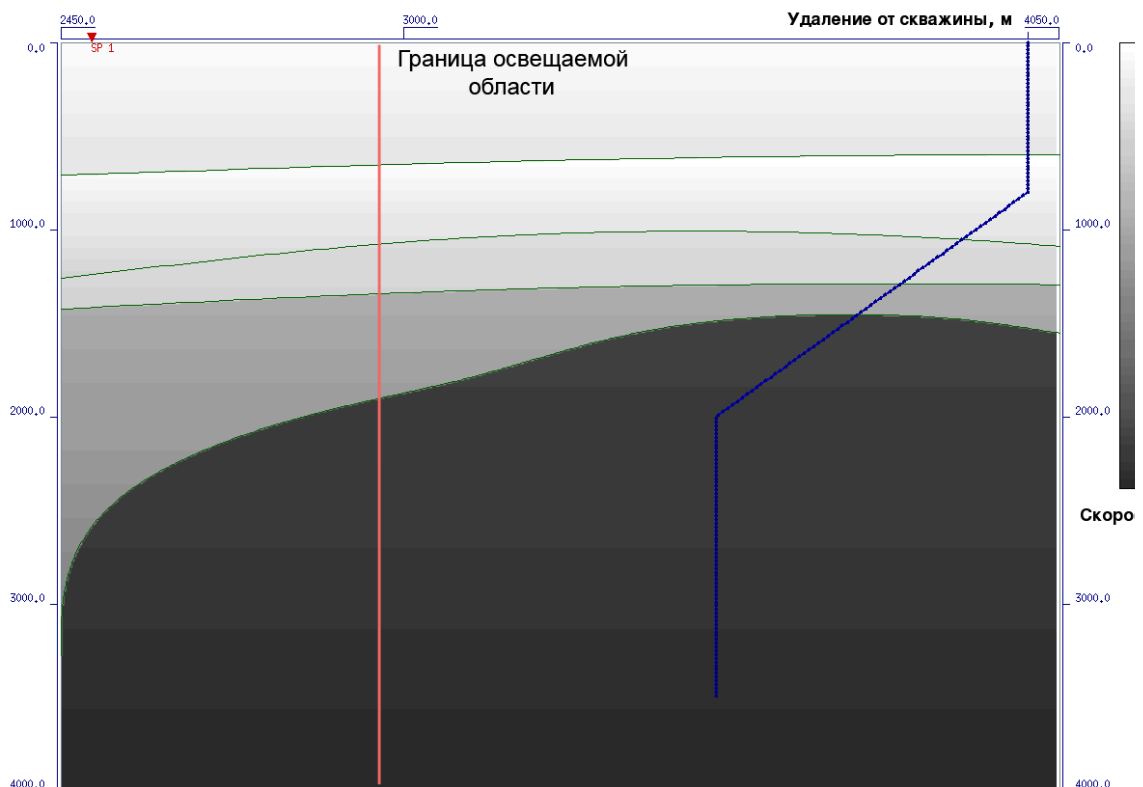
3. Результат уточнения скоростной модели среды с границами раздела пластов в виде сплайнов.
