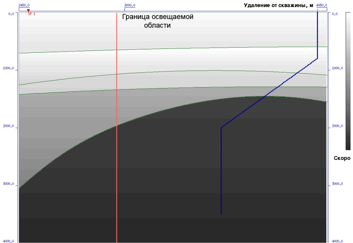
2. Результат уточнения скоростной модели среды с границами раздела пластов в виде полиномов.
